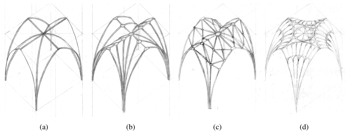
38. ábra. Csúcsíves keresztboltozat (a), sok bordás csúcsíves keresztboltozat (b), hálós boltozat (c), legyezőboltozat (d)
