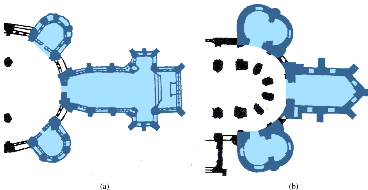
35. ábra. A gloucesteri (a) [4] és a norwichi Mária-kápolna és sugárkápolnák (b) [4]
