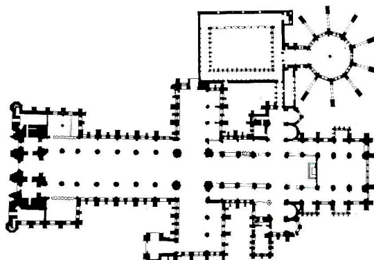
19. ábra. A lincolni katedrális alaprajza [4]
