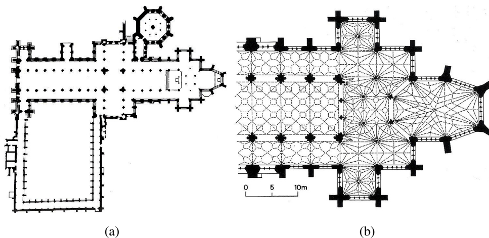
30. ábra. A wellsi katedrális alaprajza (a) [4] és a keleti végződés alaprajza a boltozatok jelölésével (b) [47]
