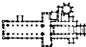
29. ábra. A southwelli katedrális alaprajza [4]
