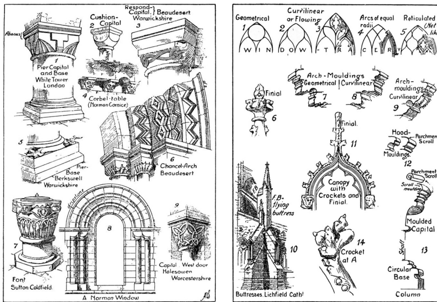
1. ábra. Részletképzések az angol gótikában [5].
