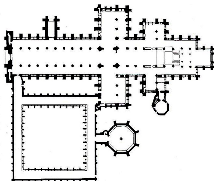
27. ábra. A salisbury-i katedrális alaprajza [4]
