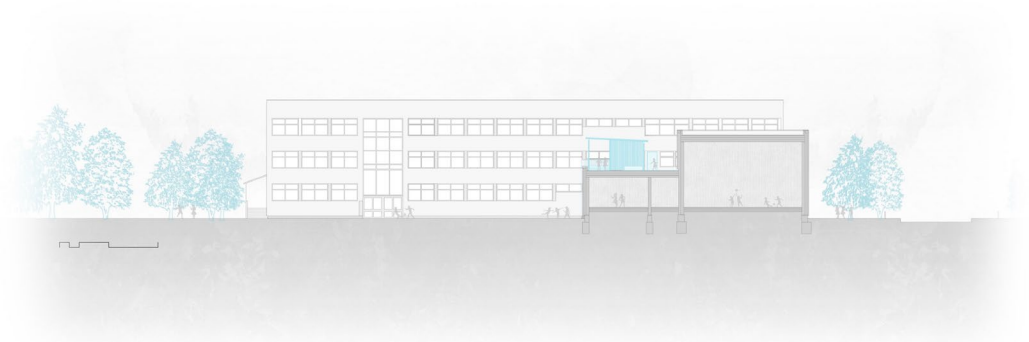
Nyugati metszet
