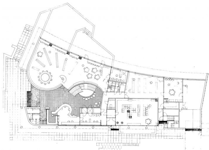
Töölö Library_ Aarne Ervi_1970_ alaprajz fsz.
