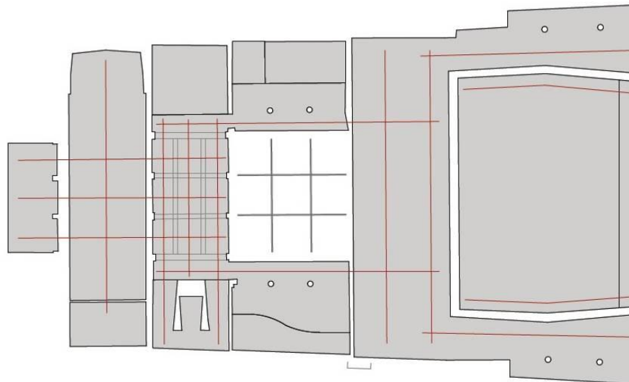
Komplex tervezés 1 Patak Gergely volt Károlyi Alajos palota Nánási Sándor terve a Rádió hangversenytermére 1966-ban, Emeleti alaprajz, M=1:200
