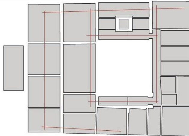
Komplex tervezés 1 Patak Gergely volt Károlyi Lajos palota Patak Gergely terve a Nemzeti Modelltár kialakítására, Földszinti alaprajz, M=1:200
