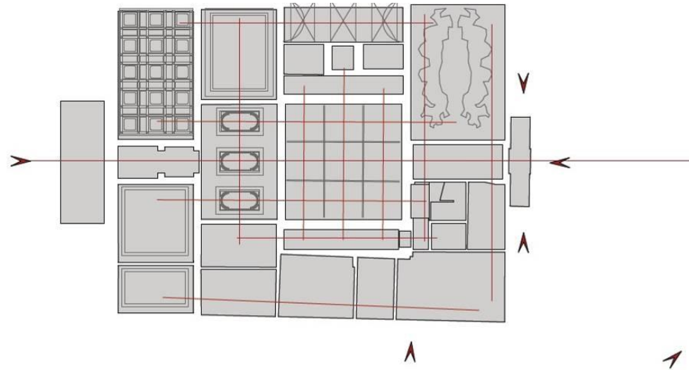
Komplex tervezés 1 Patak Gergely volt Károlyi Lajos palota Patak Gergely terve a Nemzeti Modelltár kialakítására, Földszinti alaprajz, M=1:200
