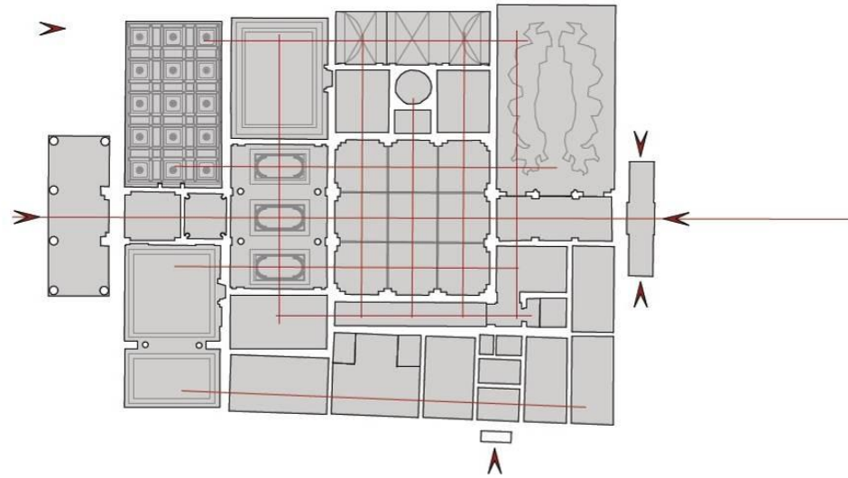
Komplex tervezés | Patak Gergely | volt Károlyi Alajos palota | 1927-es állapot, Földszinti alaprajz, M=1:200
