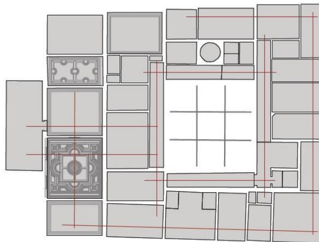
Komplex tervezés | Patak Gergely | volt Károlyi Alajos palota | 1927-es állapot, Földszinti alaprajz, M=1:200
