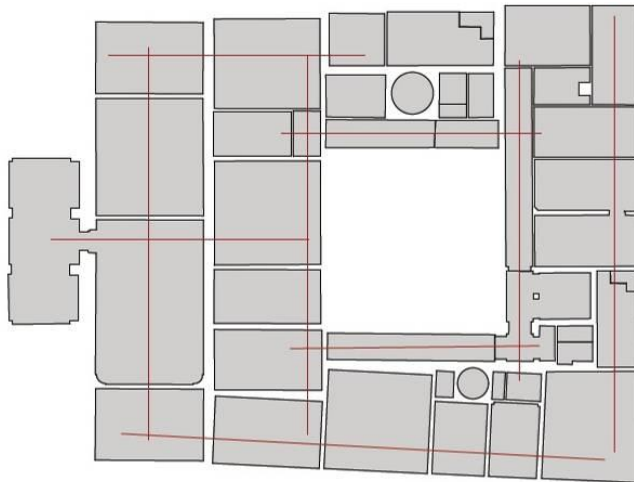
Komplex tervezés 1 Patak Gergely volt Károlyi Lajos palota Ybl Miklós 1865-ös ajánlati terve, 4. változat, I. emeleti alaprajz, M=1:200
