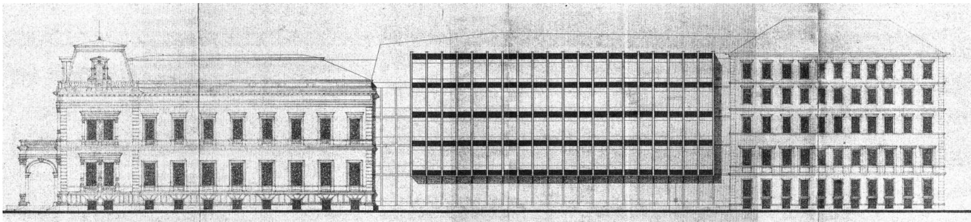
20: Magyar Rádió kiegészítő hangversenyterem terve, ÁÉTV, Nánási Sándor terve, Múzeum utcai homlokzat, 1966. december, MTVA Magyar Rádió Központi Irattára, Házgondnoksági iratok/Károlyi palota 1. doboz.
