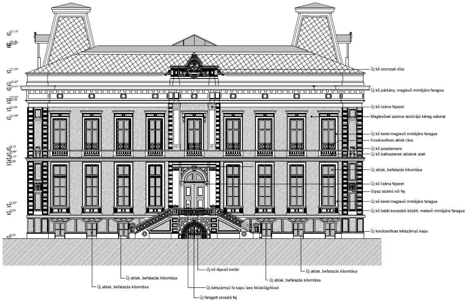
31: Csepely Knorr Kristóf terve 2010-ben, a palota kerti homlokzatának rekonstrukciójához, MTVA Magyar Rádió Központi Irattára, Házgondnoksági iratok/Károlyi palota 1. doboz.
