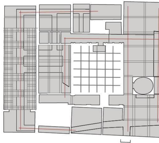
Komplex tervezés 1 Patak Gergely volt Károlyi Alajos palota 1966-os állapot, Földszinti alaprajz, M=1:200
