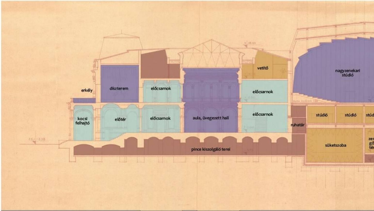
Komplex tervezés | Patak Gergely | volt Károlyi Alajos palota | Nánási Sándor terve a Rádió hangversenytermére 1966-ban, metszet, M=1:200
