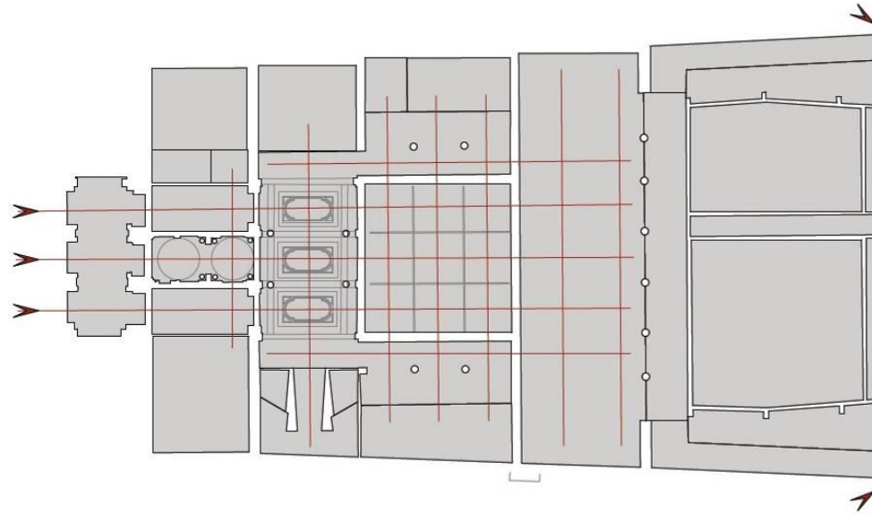
Komplex tervezés 1 Patak Gergely volt Károlyi Alajos palota Nánási Sándor terve a Rádió hangversenytermére 1966-ban, Földszinti alaprajz, M=1:200
