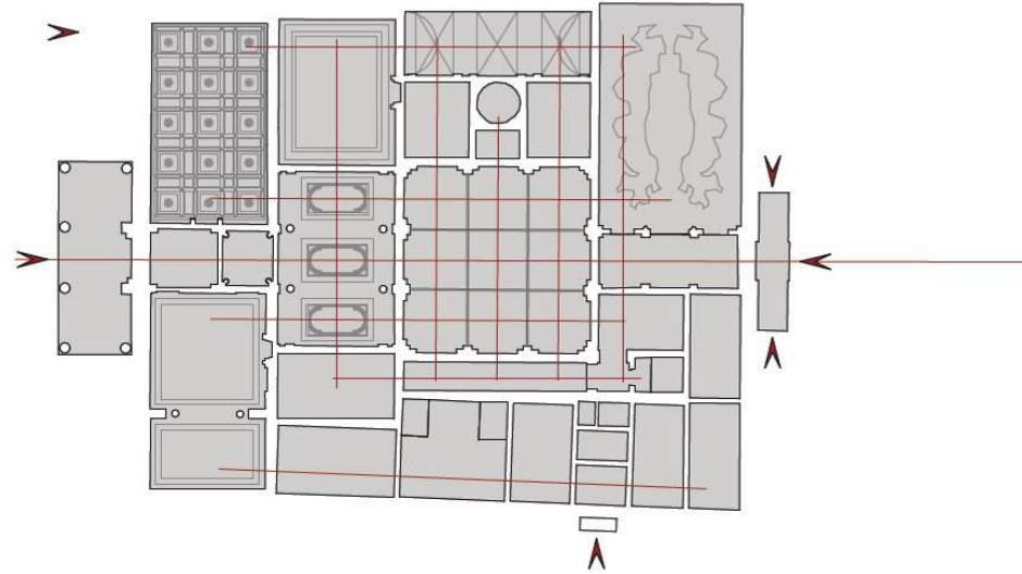
Komplex tervezés | Patak Gergely | volt Károlyi Lajos palota | 1898-as állapot, Földszinti alaprajz, M=1:200
