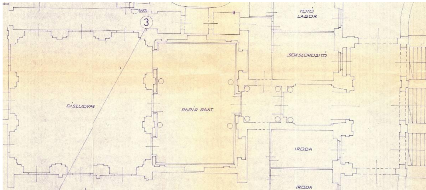
24: Fehér András földszinti átalakítási tervei, 1975. MTVA Magyar Rádió Központi Irattára, Házgondnoksági iratok/Károlyi palota 1. doboz
