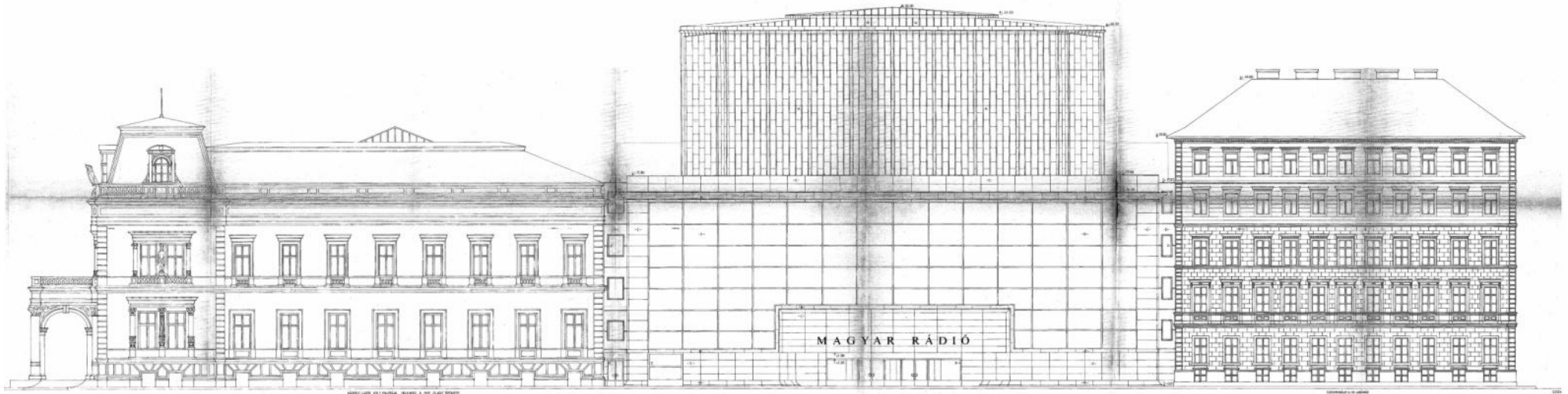
29: Gulyás Zoltán és Dobai János építészek 1987-es terve a kiegészítő hangversenystúdióra a MATERV irodán belül, MTVA Magyar Rádió Központi Irattára, Házgondnoksági iratok/Károlyi palota 1. doboz.
