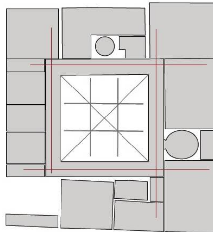
Komplex tervezés | Patak Gergely | volt Károlyi Alajos palota | Molnár Péter terve a Magyar Építőművészek Székházára 1953-ban I. emeleti alaprajz M=1:200
