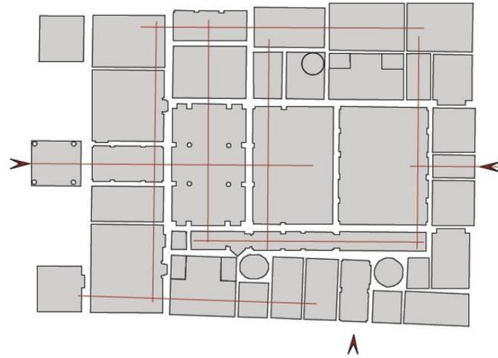
Komplex tervezés 1 Patak Gergely volt Károlyi Alajos palota Ybl Miklós 1864-es ajánlati terve, 3. változat, Földszinti alaprajz, M=1:200
