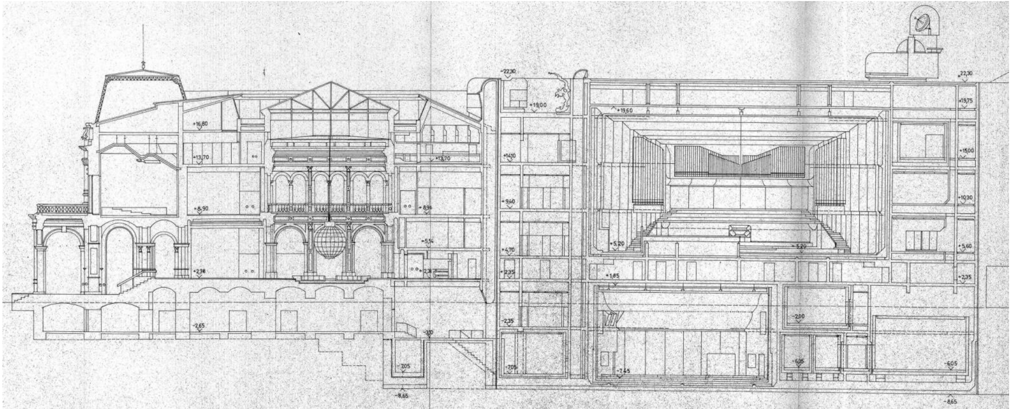
23: Gulyás Zoltán (IPARTERV) terve a kiegészítő hangversenyeremre, hosszmetset, 1973. MTVA Központi Irattár Házgondnokság iratai Károlyi palota
