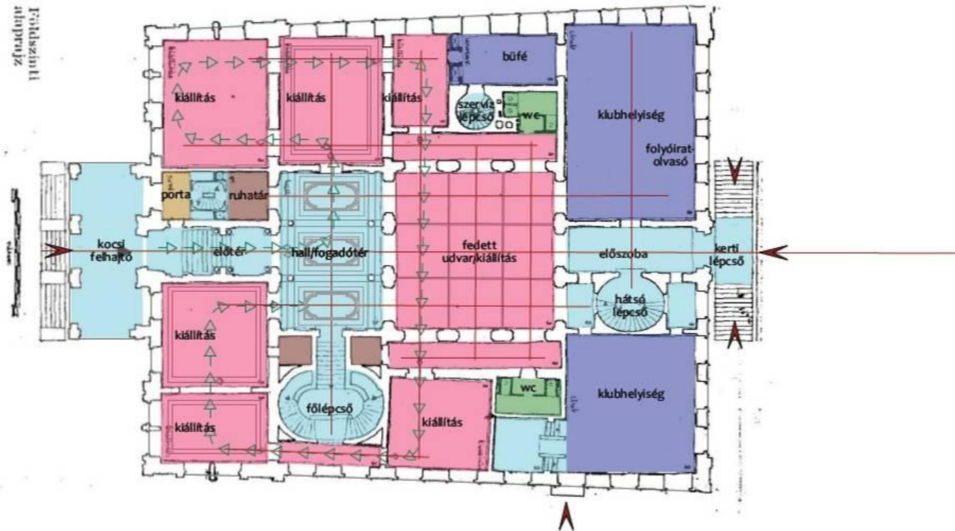
Komplex tervezés 1 Patak Gergely volt Károlyi Alajos palota Molnár Péter terve a Magyar Építőművészek Székházára 1953-ban Földszinti alaprajz M=1:200
