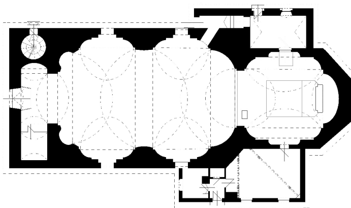
34. kép: A bagi templom alaprajza (saját rajz)
