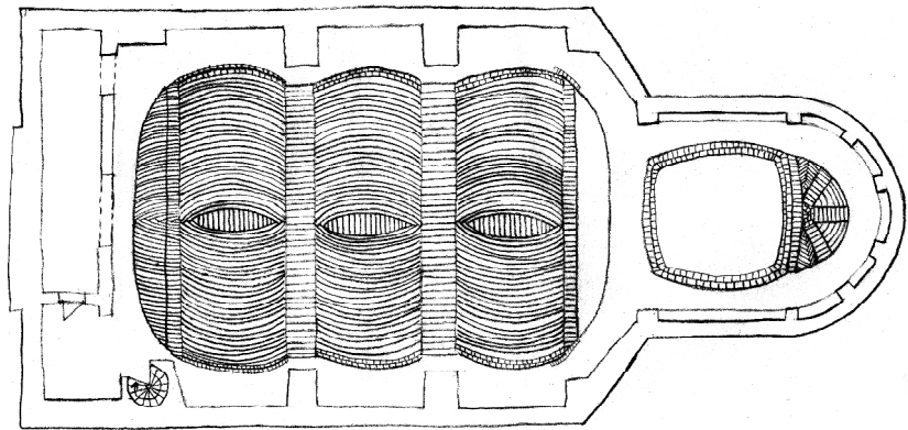
15. kép: A soroksári templom boltozata (saját rajz)
