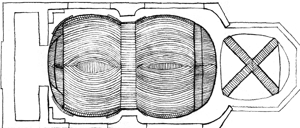
41. kép: A boldogi templom boltozata (saját rajz)
